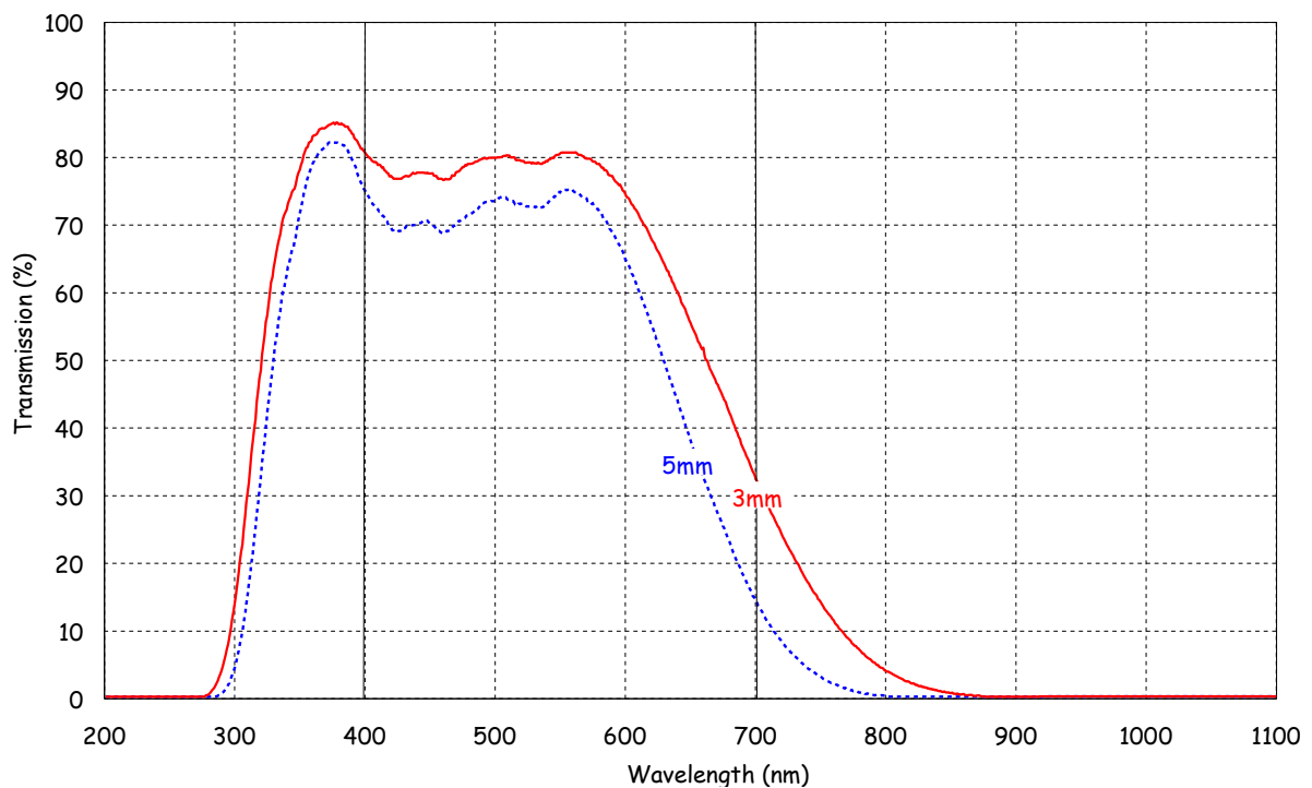
Curva di Trasmissione E233 (eq KG3)
