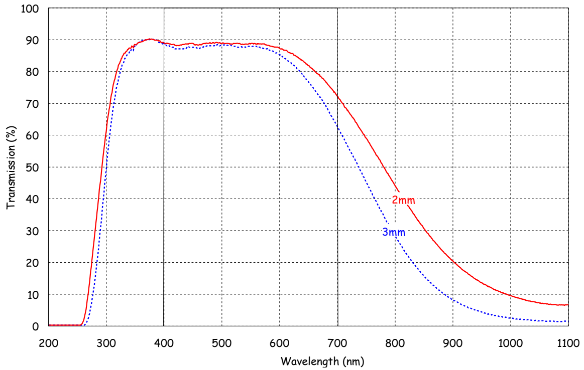
Curva di Trasmissione E231 (eq KG1)
